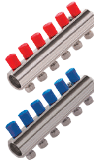
► Vanalı Kollektör - Pirinç 1 1/4"-16x2 (PN 10)
