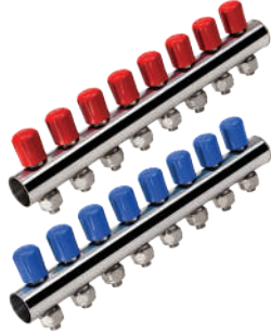
► Vanalı Kollektör - Paslanmaz Çelik 1"-16x2 (PN 10)
