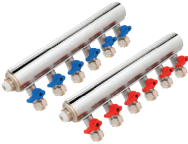
► 3/8 Mini Vanalı Kollektör - Pirinç 1"-16x2 (PN 10)
